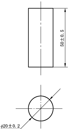
图 1 抗压强度试件成型模具
