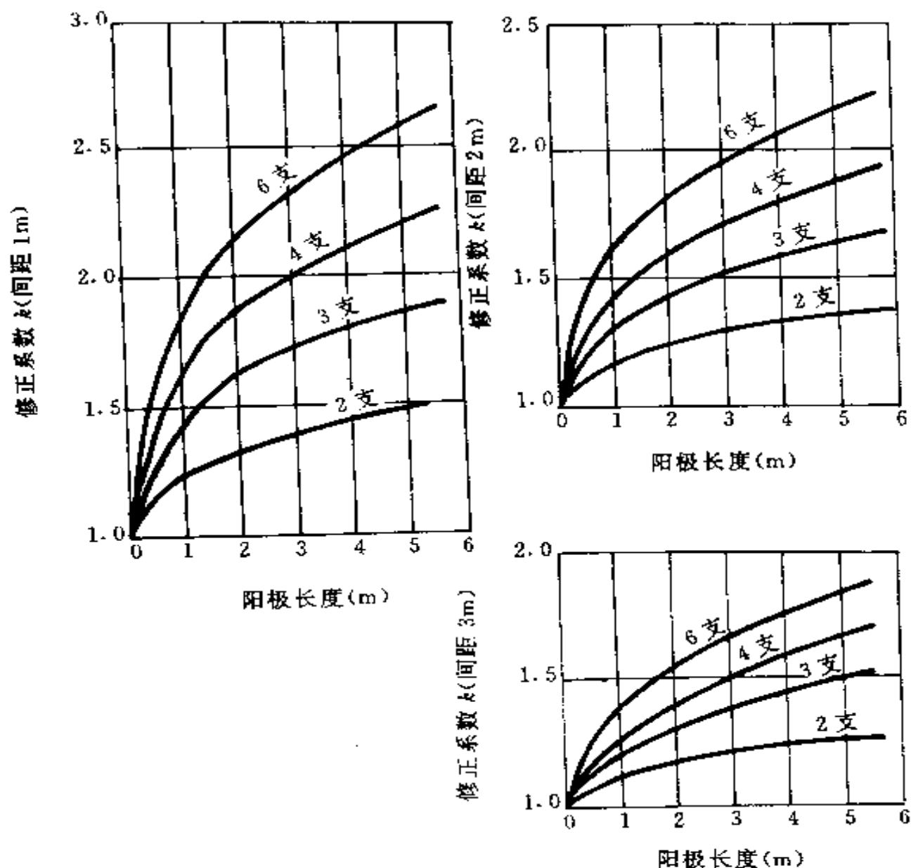
图 5.0.2 阳极接地电阻修正系数 k
