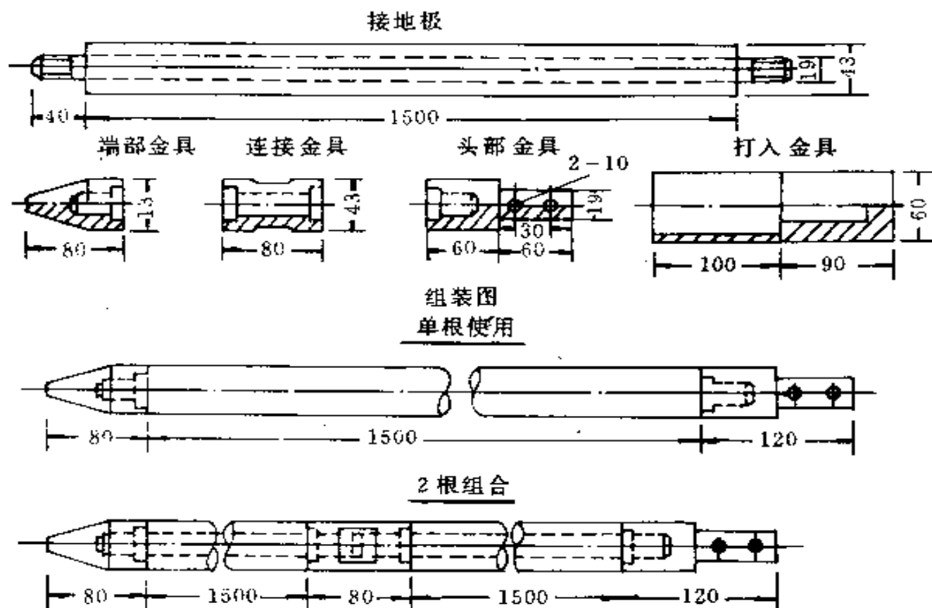
图 4.2.5 锌接地极结构图
