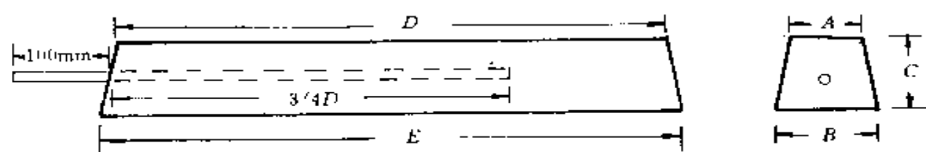
梯形截面镁阳极形状及尺寸
