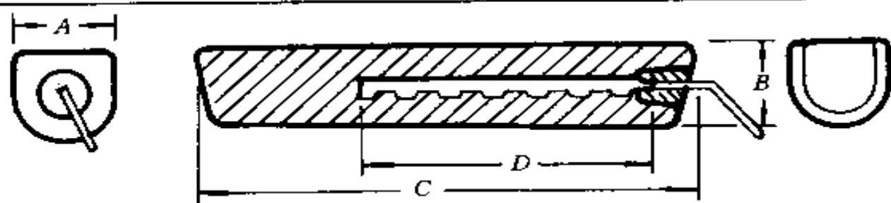
D 形截面镁阳极形状及尺寸
